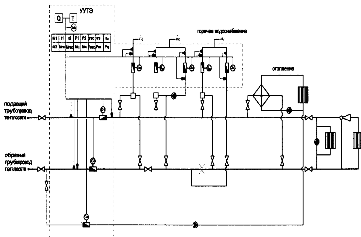
Рис. 6. Варианты принципиальной схемы размещения точек измерения количества тепловой энергии и массы (объема) теплоносителя, а также его регистрируемых параметров в открытых системах теплоснабжения (PT - регулятор температуры).
